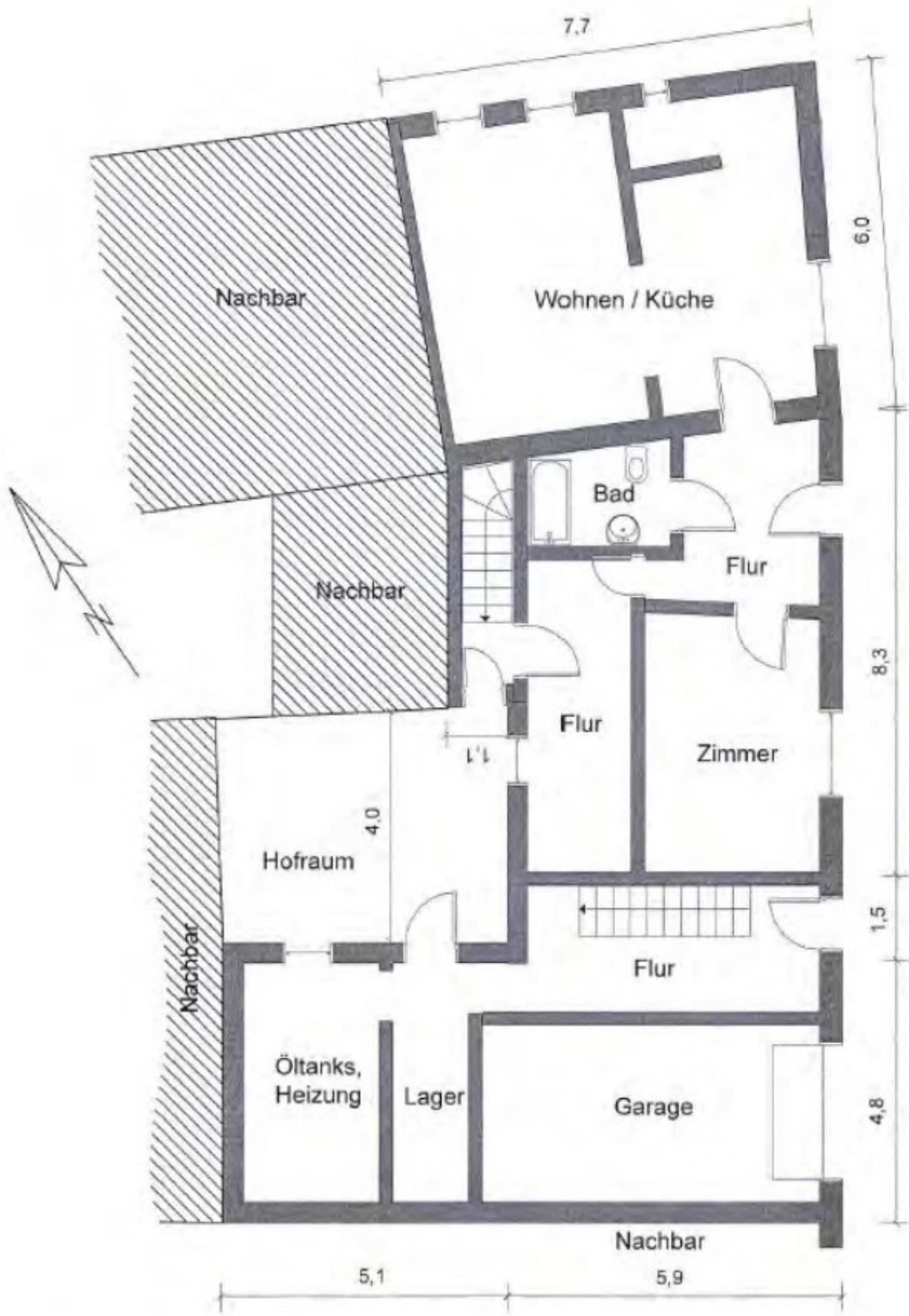
Skizze Erdgeschoss
